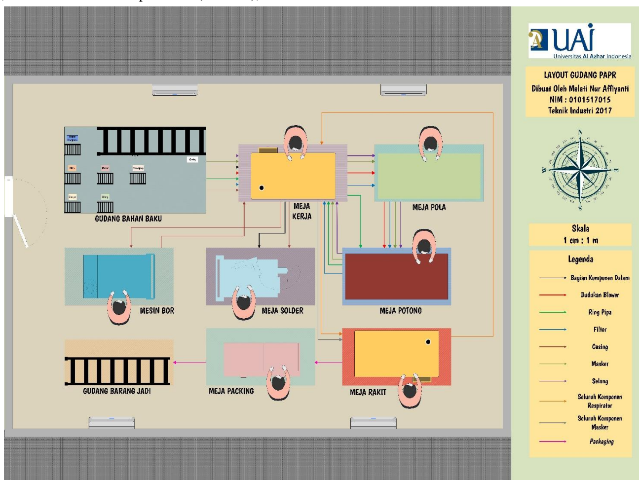
Gambar 5. Layout Lantai Produksi LCC RESPIRA V.01
