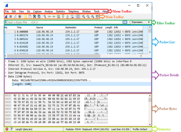
Gambar 5. Struktur Wireshark
