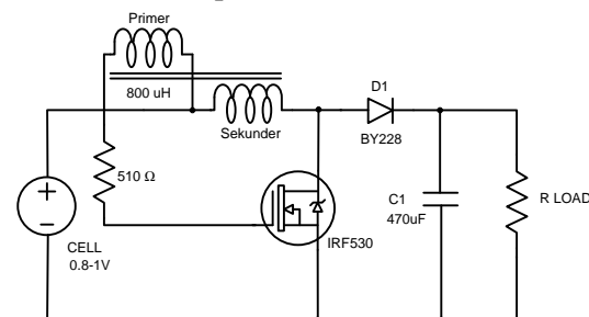
Gambar 4. Siruit dari boost converter hasil penelitian
